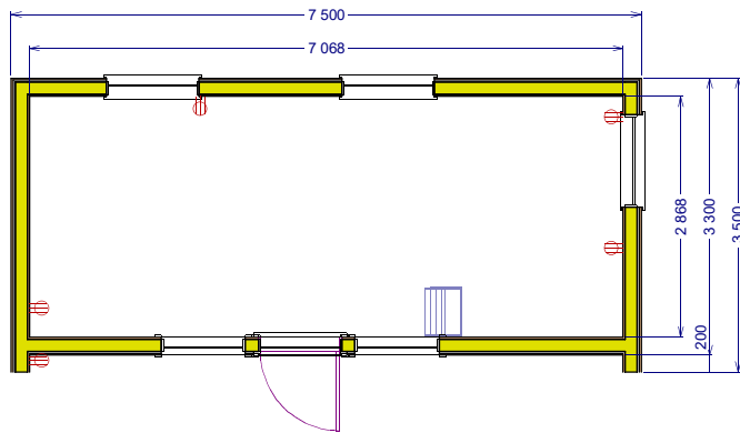
Plan 1, entréplan
