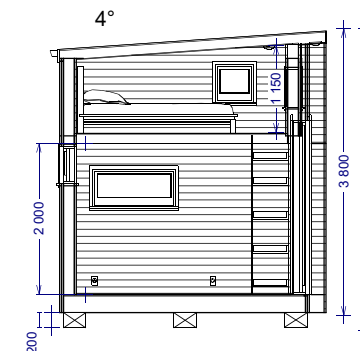
Sektion, a-a
