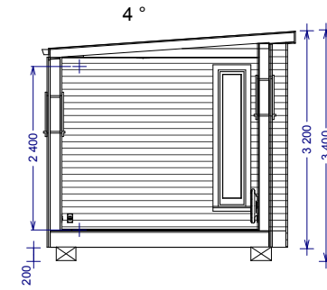
SEKTION
