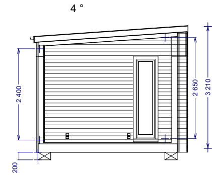
SEKTION
